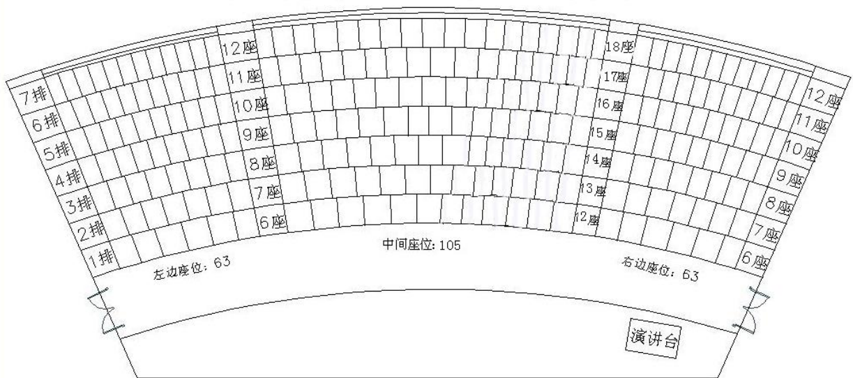
国际会议中心139报告厅平面图
